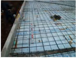
侑ハウス作業棟新築工事 107
